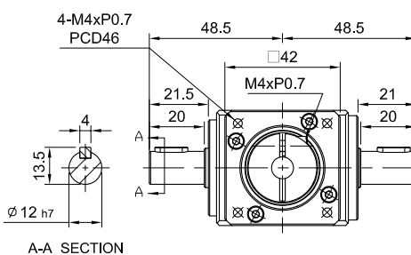
A-A SECTION
