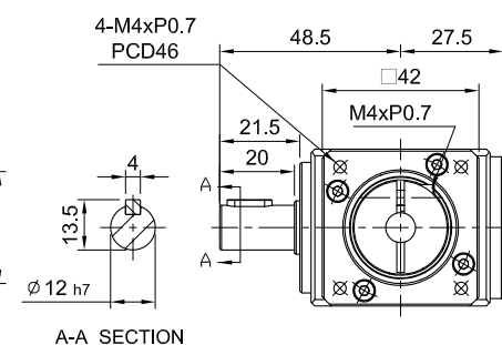
A-A SECTION
