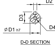
D-D SECTION
